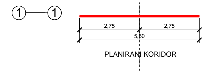
POPREČNI PROFIL M 1 : 100
